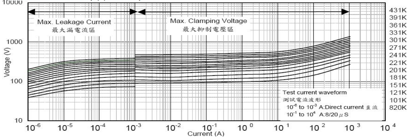
VDR-14D820K-14D431K(N/J/S SERIES)
