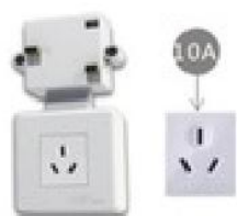
移动单插座（220V/10A） 型号：HGS-YC(1P10) 物料编码：01091301
