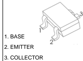
SOT-323
