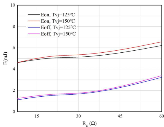
图 5. 开关损耗
