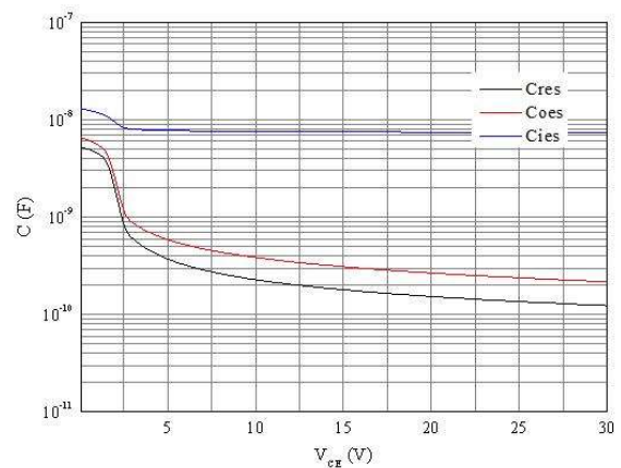
图 6. 电容特性
