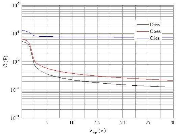
图 11. 电容特性
