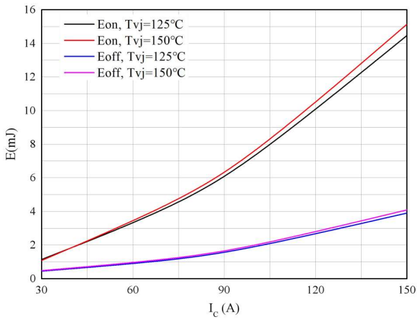
图 7. 开关损耗
