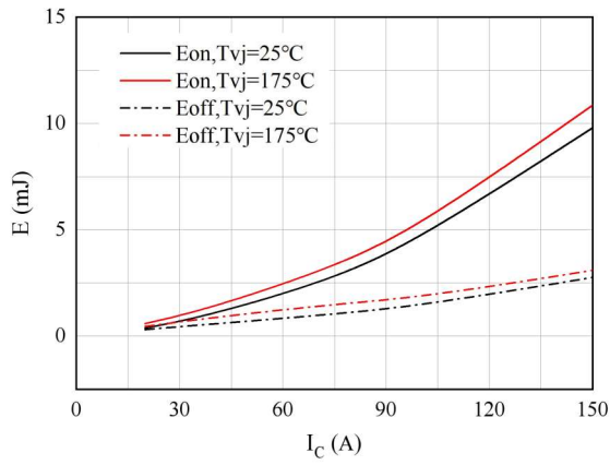
图 7. 开关损耗
