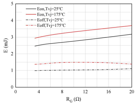
图 8. 开关损耗
