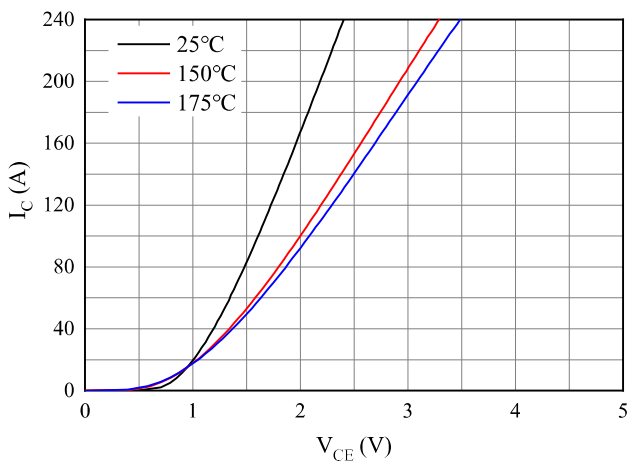
图 3. 典型输出特性 ( V_{GS}=15\text{V} )
