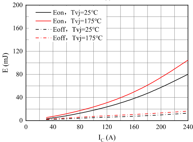
图 9. 开关损耗
