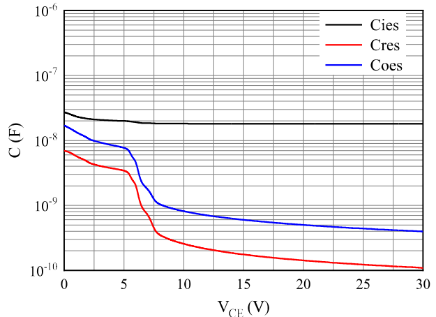
图 6. 电容特性
