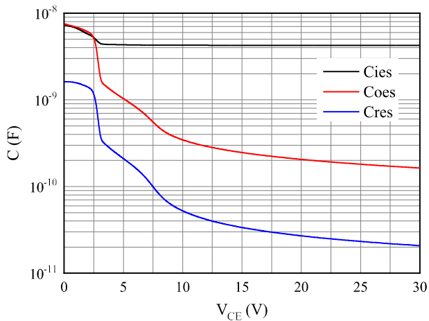
图 11. 电容特性
