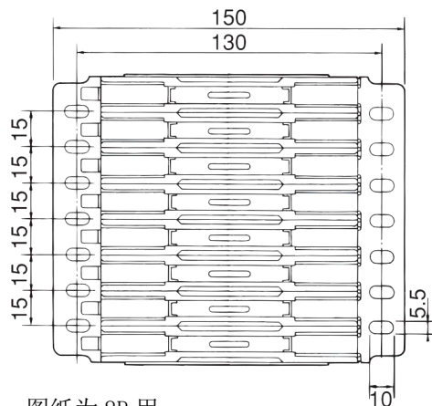
图纸为 8P 用
