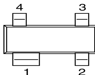
SOT143
